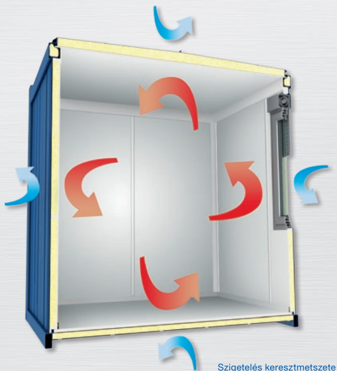
Szigetelés keresztmetszete
